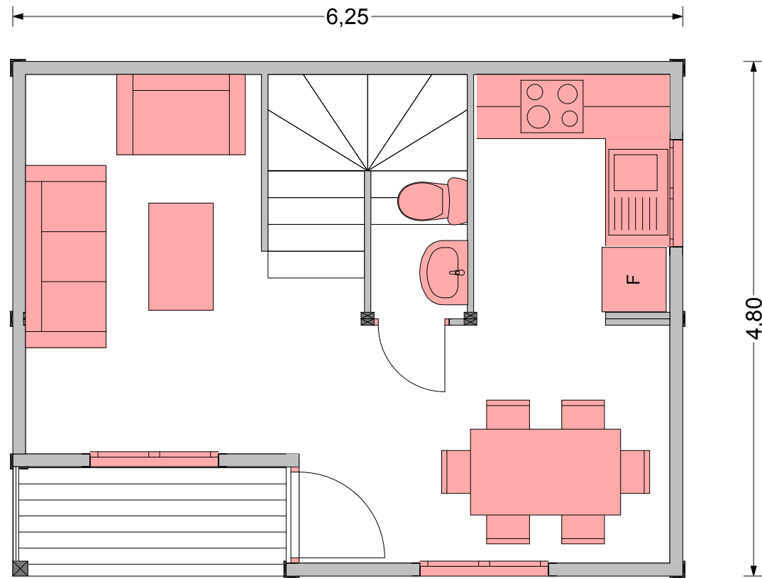
modelo BILOBA 60 planta baja
