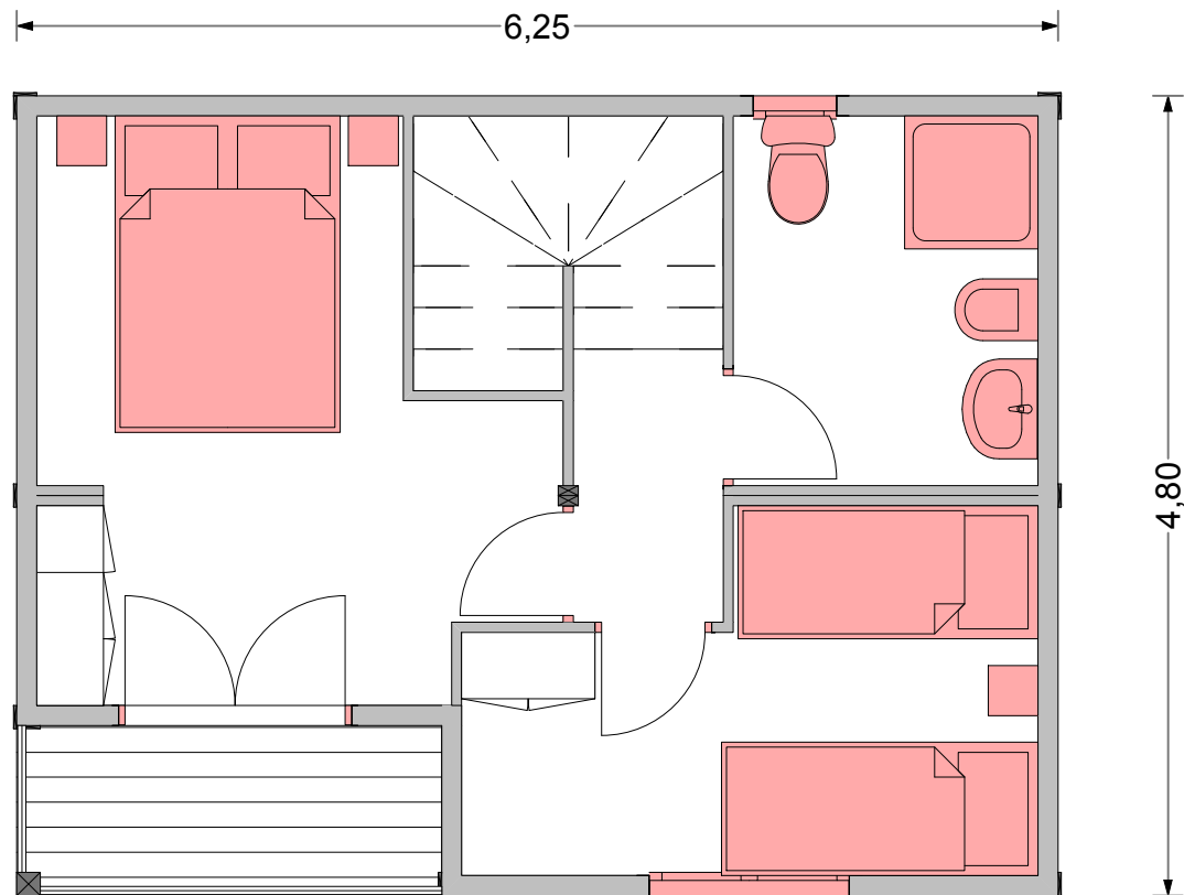
modelo BILOBA 60 planta superior www.casascarbonell.com
