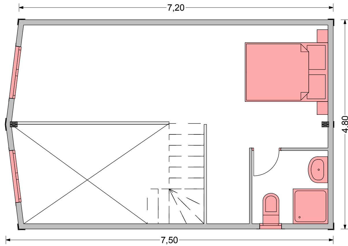
modelo PERAL 70 PLANTA SUPERIOR
