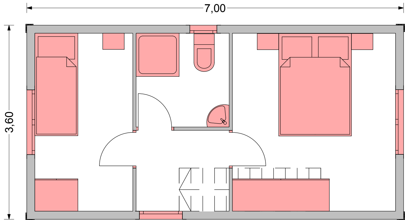
modelo ALCOY 50 planta 1 www.casascarbonell.es
