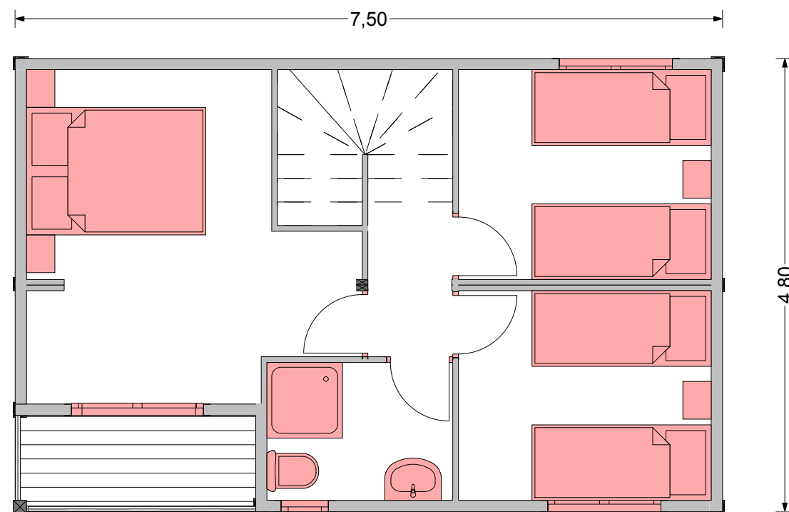
modelo GUAYABA 72 1ª planta
