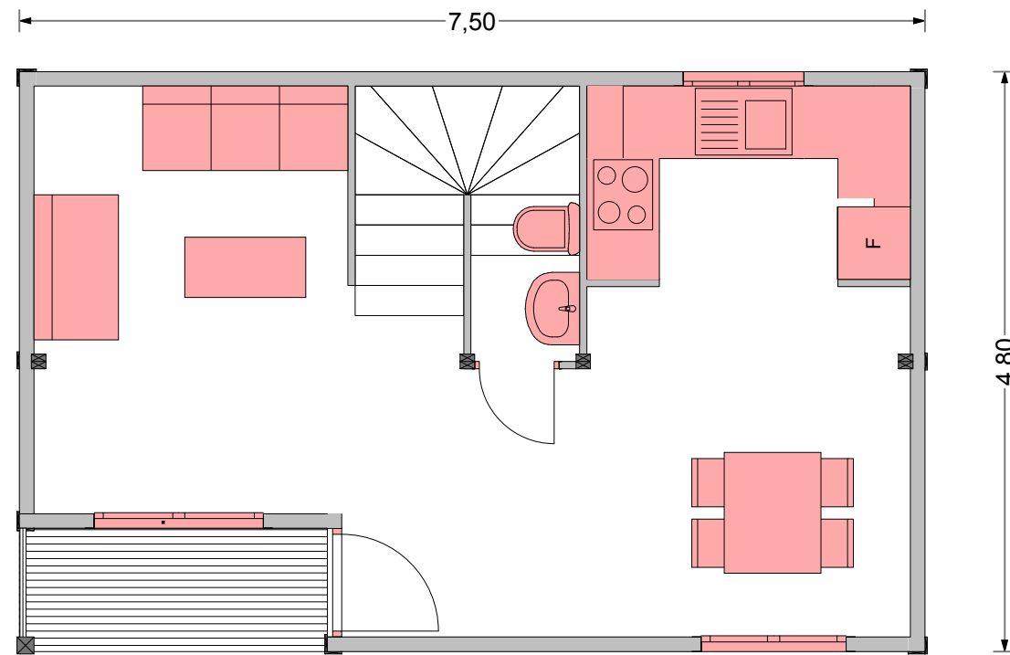
modelo GUAYABA 72 planta baja
