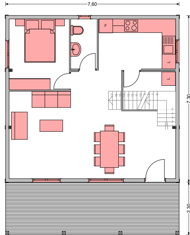
modelo Sagunto 138 planta baja
