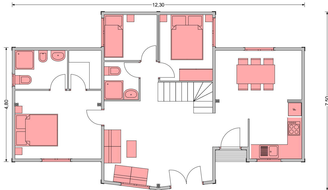
modelo ACACIA PLANTA INFERIOR
