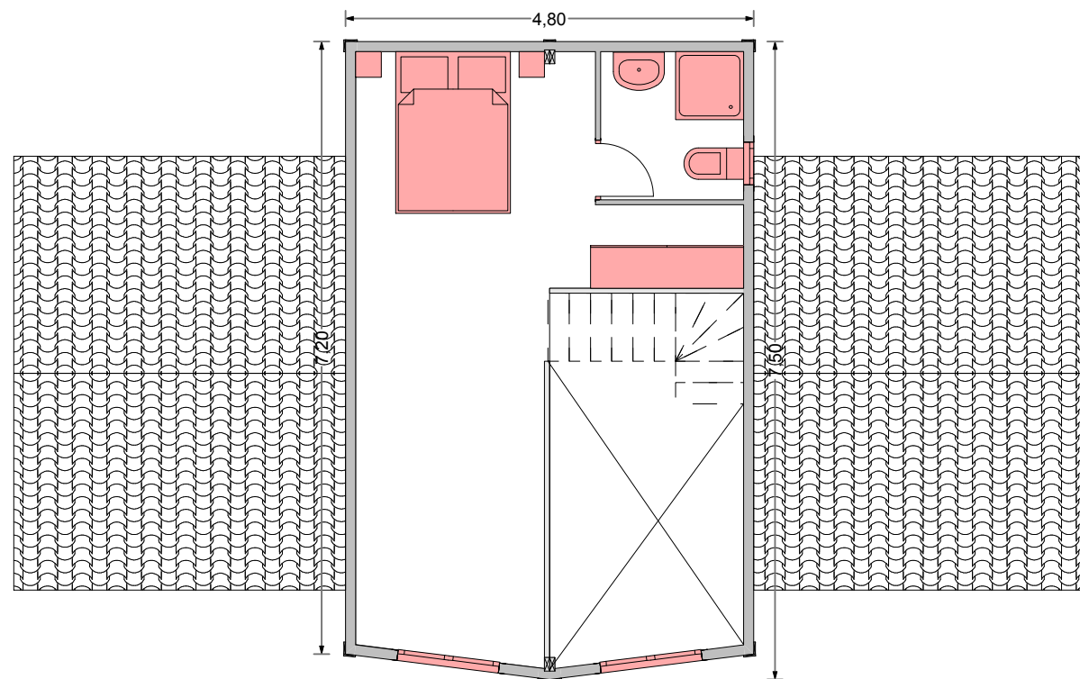
modelo ACACIA 106 PLANTA SUPERIOR
